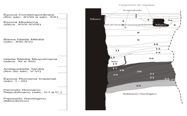
Fig. 4 - Corte estratigráfico da intervenção, com os contextos romanos assinalados a cinza.
